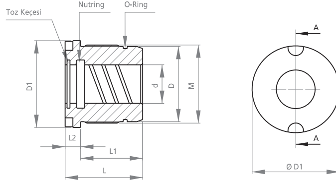
KESİT(SECT.) A-A
